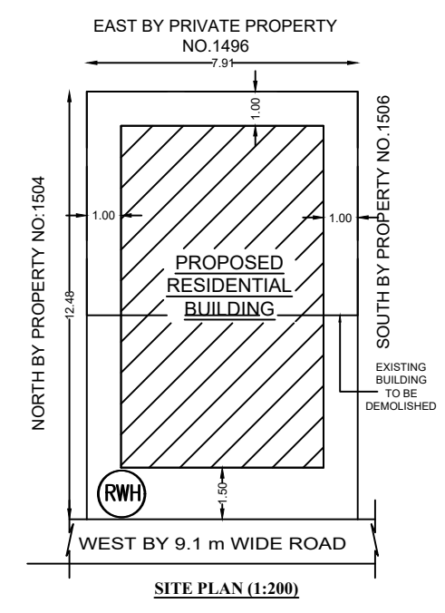
SITE PLAN (1:200)
